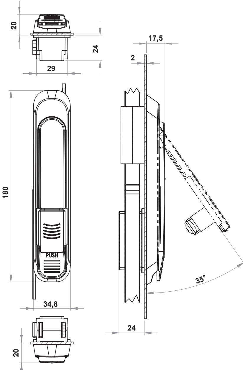
2307 - Basmalı Tip Kollu Kilit (Kol zamak, siyah boyalı, gövde plastik)
