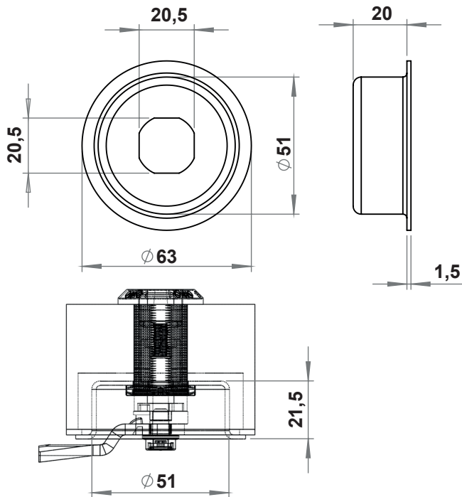
2900-450 - Montaj Sacı
