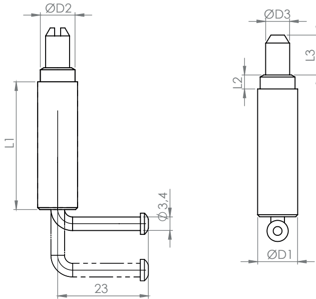
3028 - 120° Mentşe
