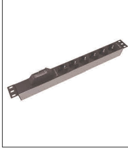
PDU - 19" 1U Enerji Ölçerli (kWh aktif enerji)
