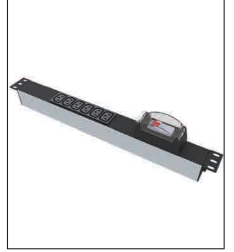
PDU - 19" 1U IEC320 C13 prizli Sigortalı (1P)
